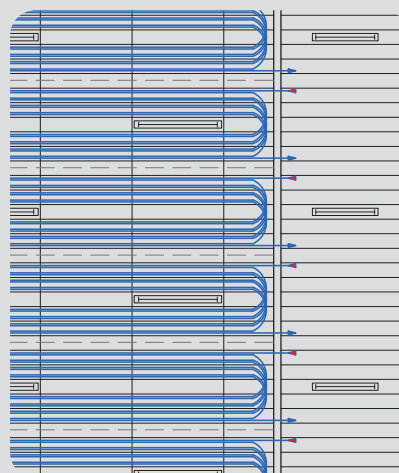
Circuito soffitto metallico EASY-KLIMA®
