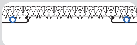
1. Struttura appesa dotata di sistema di aggancio rapido
