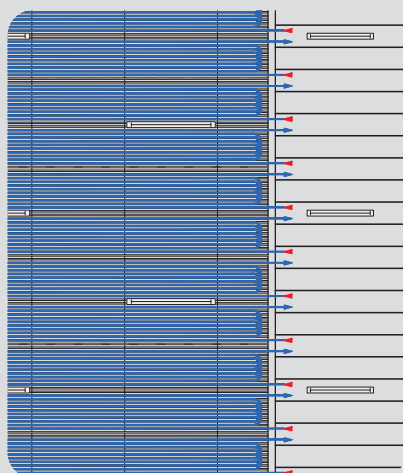
Circuito soffitto metallico SAPP®
