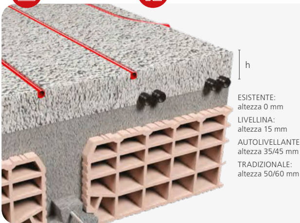
altezza del sistema esclusa finitura. Gli spessori sono indicativi, possono variare in base al prodotto usato
