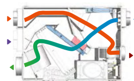
Flusso free cooling
