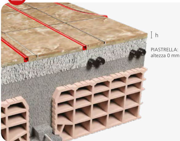
altezza del sistema esclusa finitura
