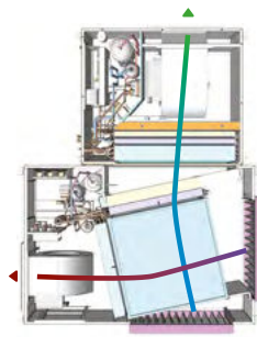
Flusso ricircolo, ricambio e trattamento aria
