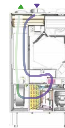
Flusso ricircolo e trattamento aria
