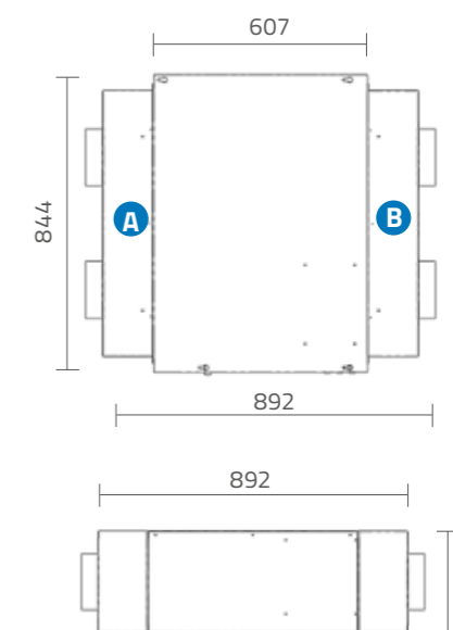
A. Immissione aria trattata, 2x \phi 160* B. Ripresa aria locali puliti, 2x \phi 160*
