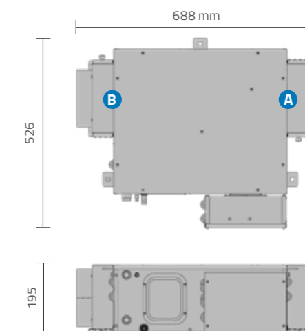
A. Immissione aria trattata, ø 160 B. Ripresa aria locali puliti, ø 160
