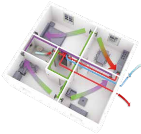
Flusso ricircolo e trattamento aria
