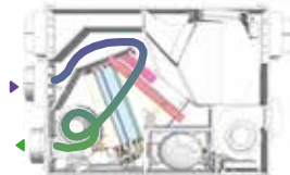
Flusso ricircolo e trattamento aria
