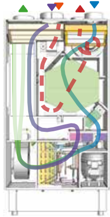
Flusso ricircolo, ricambio e trattamento aria
