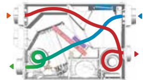
Flusso free cooling
