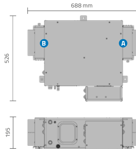
A. Immissione aria trattata, \varnothing 160 B. Ripresa aria locali puliti, \varnothing 160
