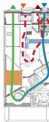
Flusso free cooling
