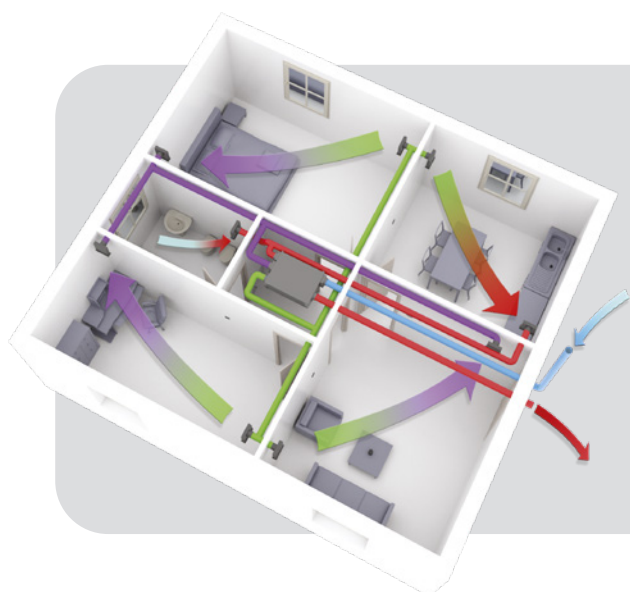
Flusso ricambio dell'aria
