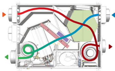
Flusso ricambio dell'aria
