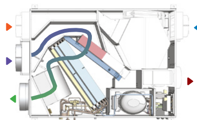
Flusso ricircolo e trattamento aria
