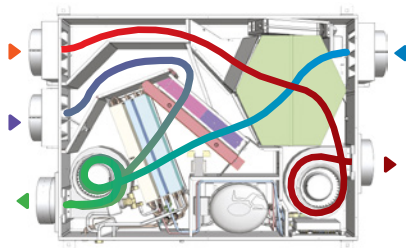
Flusso ricircolo, ricambio e trattamento aria
