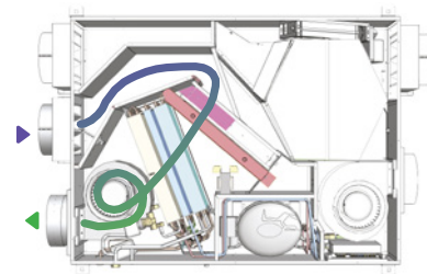
Flusso ricircolo e trattamento aria
