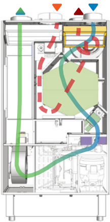
Flusso ricambio dell'aria
