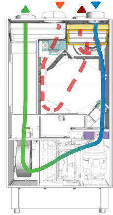
Flusso free cooling
