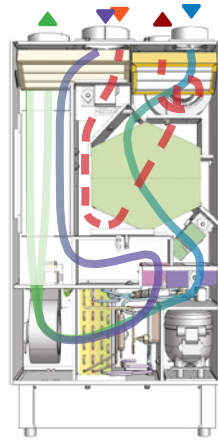
Flusso ricircolo, ricambio e trattamento aria
