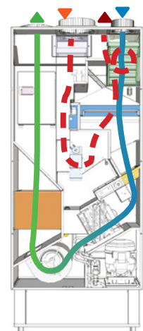
Flusso free cooling
